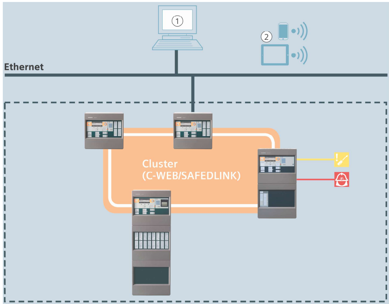
Fig. 2: Sub-net
